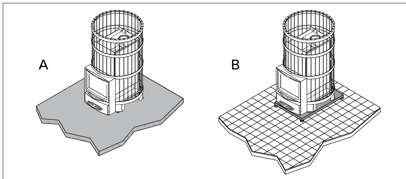
Kuva 8. Lattian suojaaminen (mitat millimetreinä) Bild 8. Skydd av golvet (måttan i millimeter)
