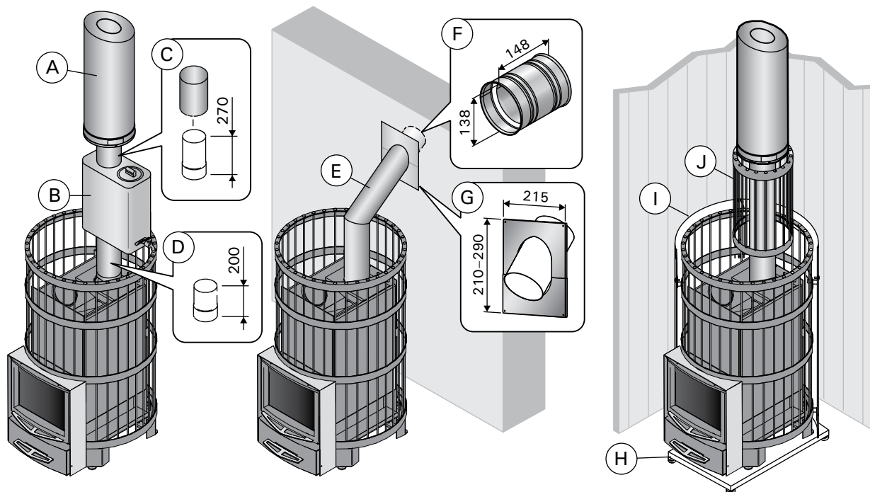
Figure 16. Accessoires (toutes les dimensions sont fournies en millimètres)
