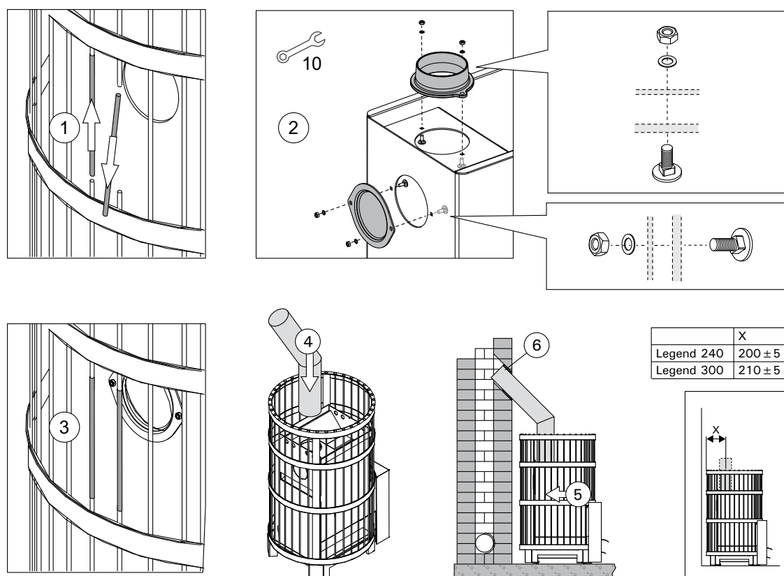
Figure 12. Raccordement du poêle à un conduit maçonné via l'ouverture de raccordement supérieure (toutes les dimensions sont fournies en millimètres)
