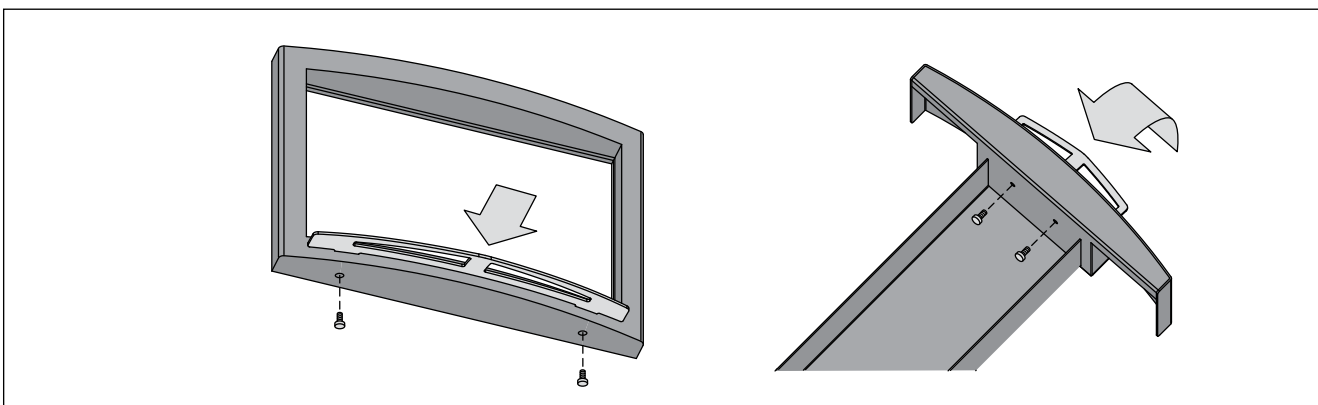
Рисунок 15. Установка рукояток Joonis 15. Käepidemete paigaldamine
