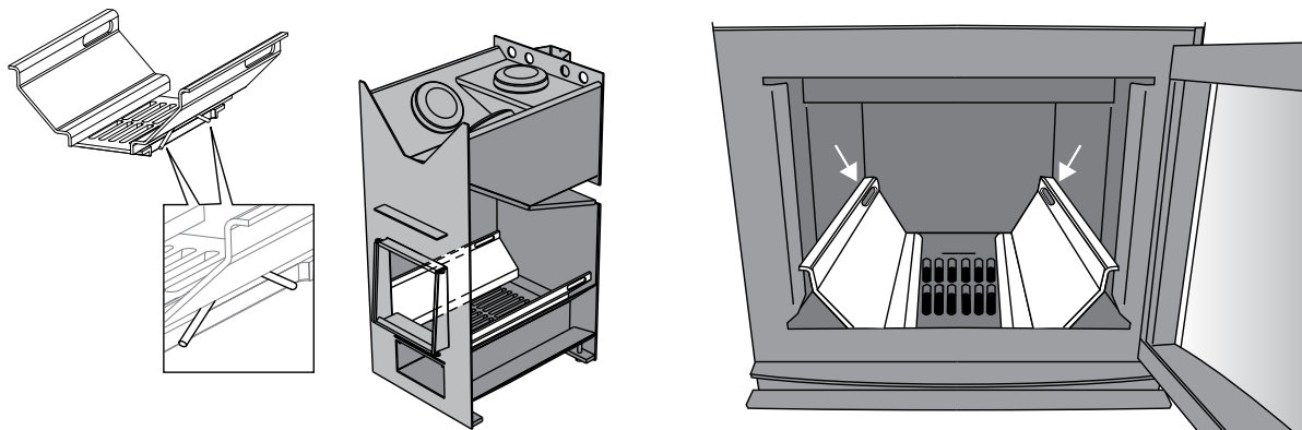
Рисунок 2. Каналы для подачи воздуха для горения Joonis 2. Põlemiskambri õhukanalid
