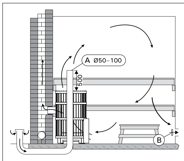
Figure 7. Ventilation meccanica Figura 7. Sistema di ventilazione meccanico
