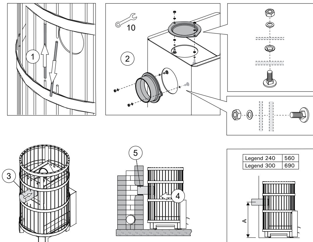
Figure 11. Raccordement du poêle à un conduit maçonné via l'ouverture de raccordement arrière (toutes les dimensions sont fournies en millimètres)
