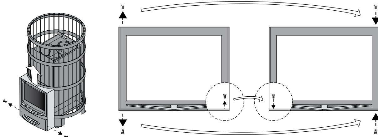
Kuva 14. Luukun käsisyyden vaihtaminen Bild 14. Byte av luckans öppningsriktning
