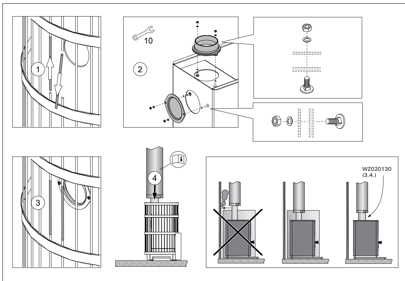
Kuva 13. Kiukaan liittäminen Harvia-teräspiippuun
