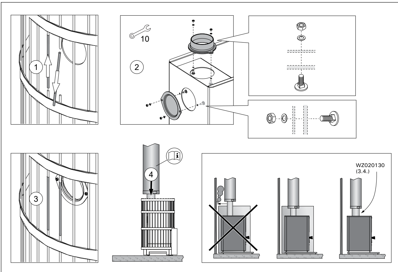
Kuva 13. Присоединение печи к стальному дымоходу Harvia Bild 13. Kerise ühendamine Harvia teraskorstnaga
