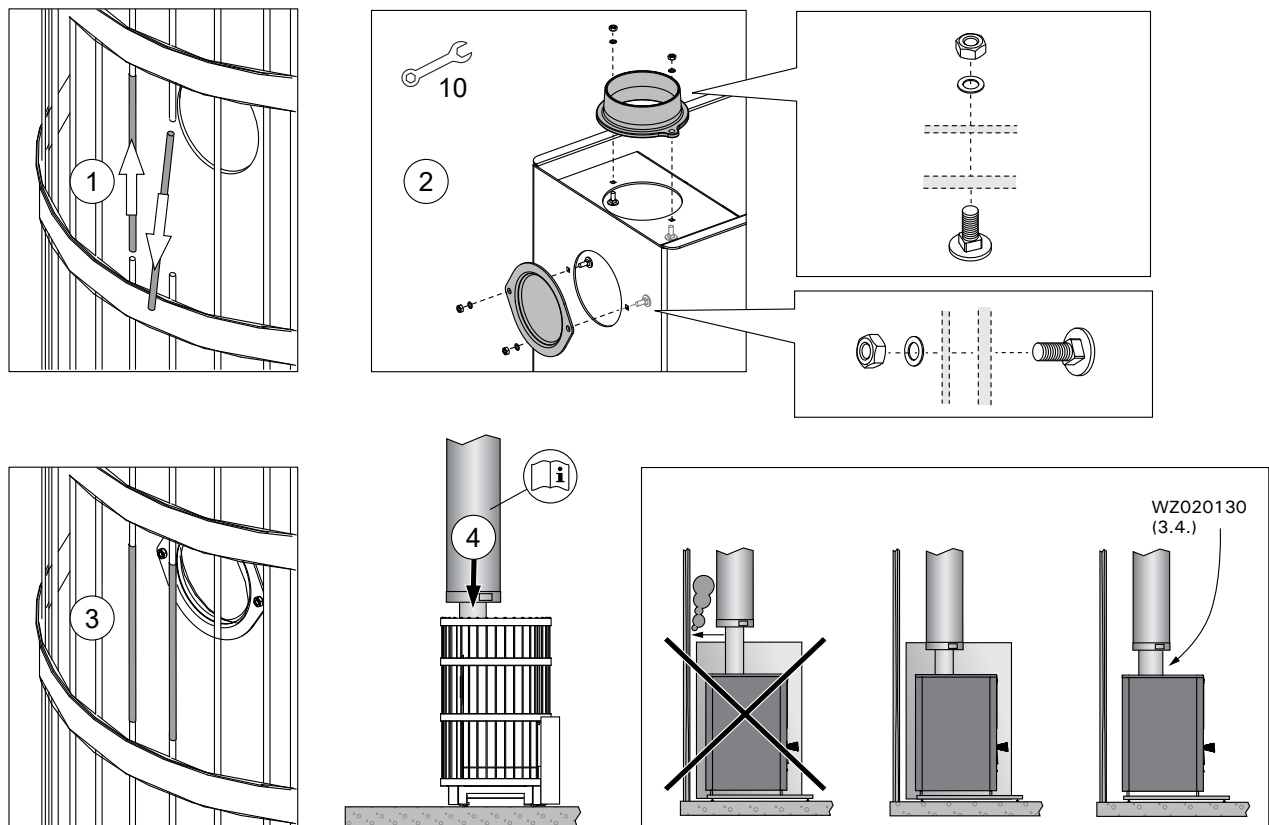
Kuva 13. De kachel aansluiten op een stalen schoorsteen van Harvia
