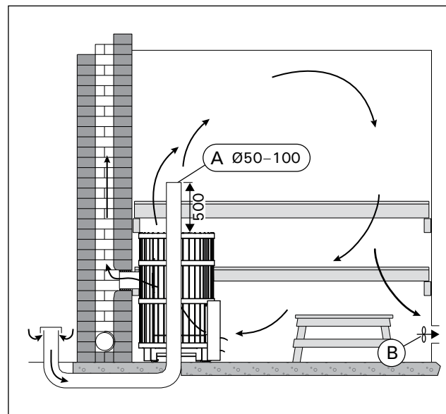
Kuva 7. Koneellinen ilmanvaihto Bild 7. Maskinell ventilation
