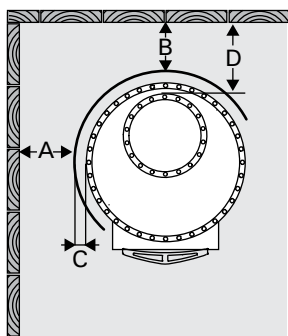
Рисунок 10 Элементы защиты Legend Joonis 10. Legend kaitsetarvikud
