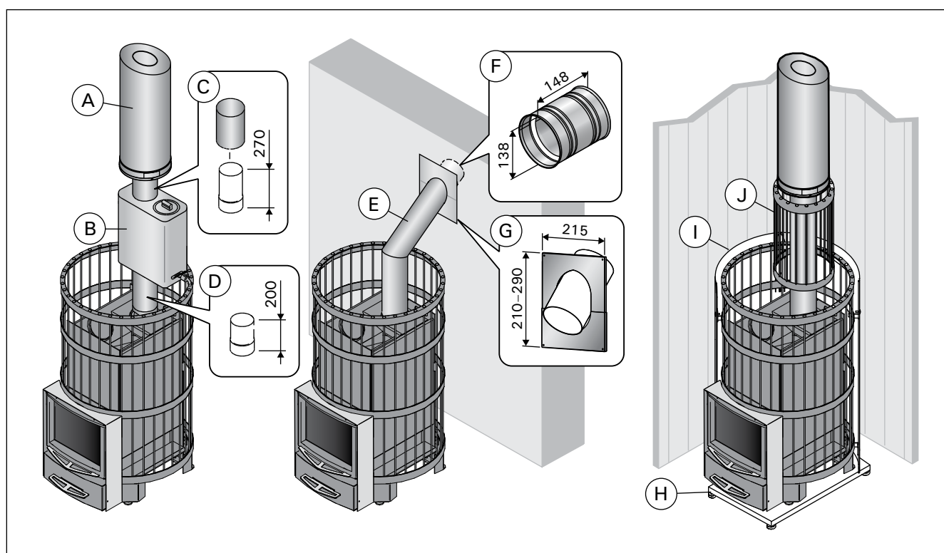
Figuur 16. Accessoires (alle afmetingen in millimeters)
