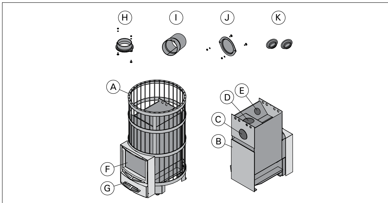
Kuva 1. Kiukaan osat. Huom! Kiukaaseen ei saa tehdä muutoksia ilman valmistajan suostumusta.
