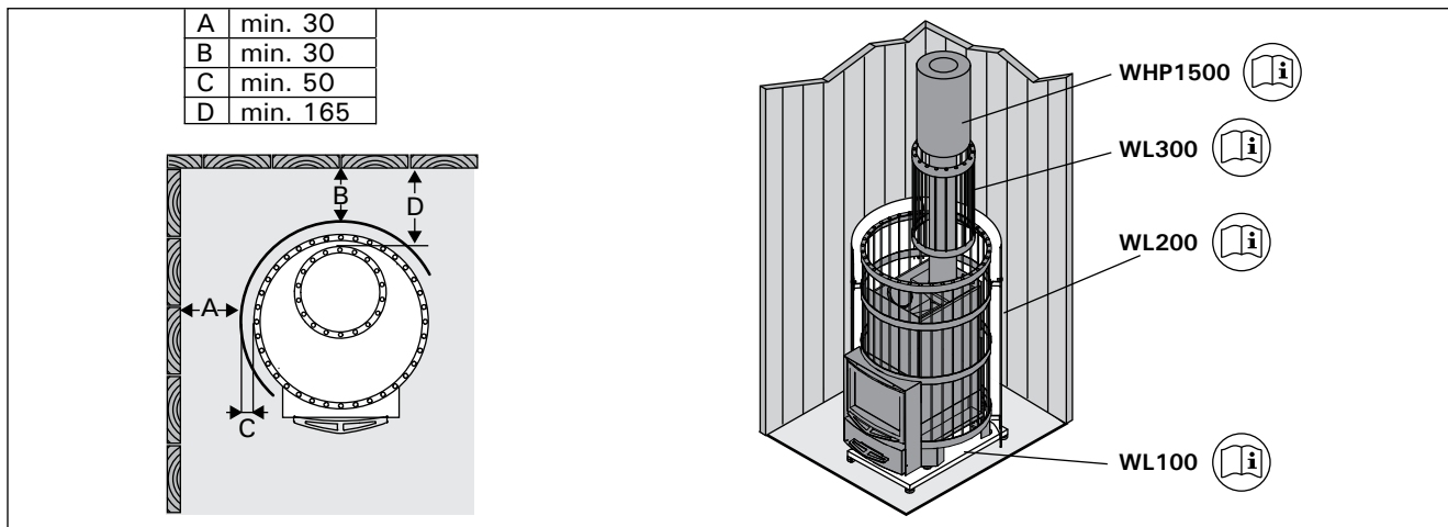
Kuva 10. Legend-suojaustarvikkeet (mitat millimetreinä)
