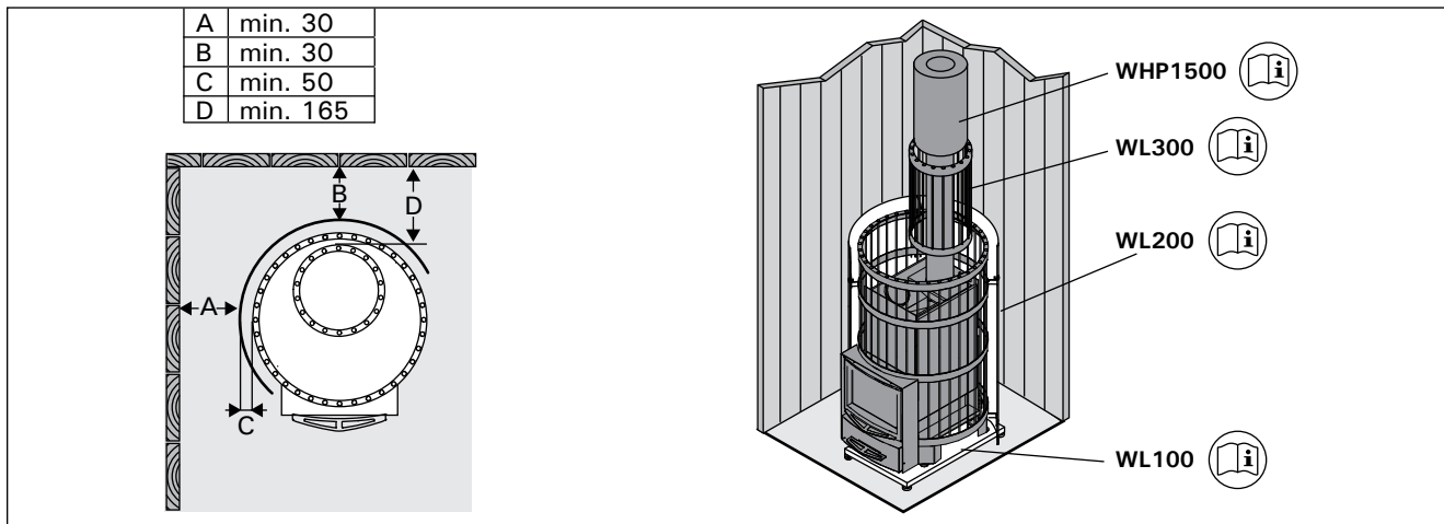
Figure 10. Legend Protections (toutes les dimensions sont fournies en millimètres) Figura 10. Legend Dispositivi di protezione (tutte le dimensioni sono espresse in millimetri)
